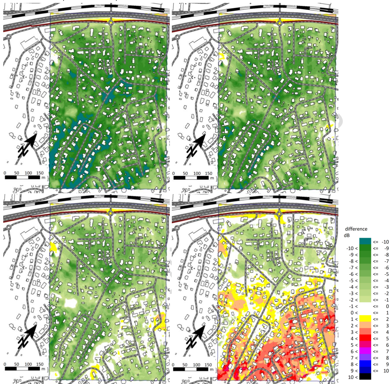
Figur 41. Lerum, villaområde, skillnadsplottar ( L_{AFmax} ) Nord2000 – Nord96, beräkningshöjd = 2 m.
