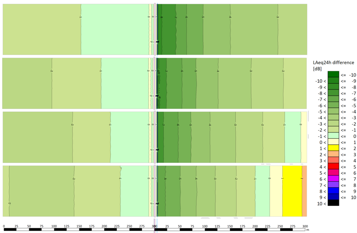
Figur 11. Skillnadsplottar ( L_{Aeq24h} ) Nord2000 – Nord96, beräkningshöjd = 2 m, höjd banvall = 0,5 m, hård mark. Vindhastighet uppifrån: 1 m/s, 1,5 m/s, 2 m/s och 3 m/s.
