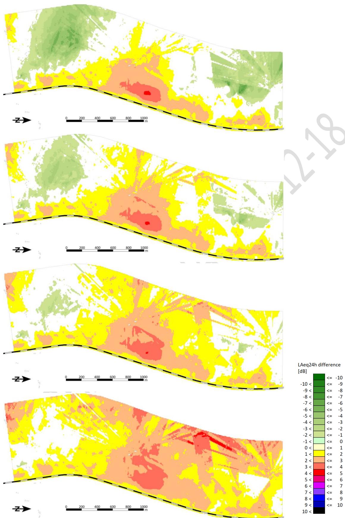
Figur 46. Västerås, skillnadsplottar ( L_{Aeq24h} ) Nord2000 – Nord96, beräkningshöjd = 8 m. Vindhastighet uppifrån: 1 m/s, 1,5 m/s, 2 m/s och 3 m/s.
