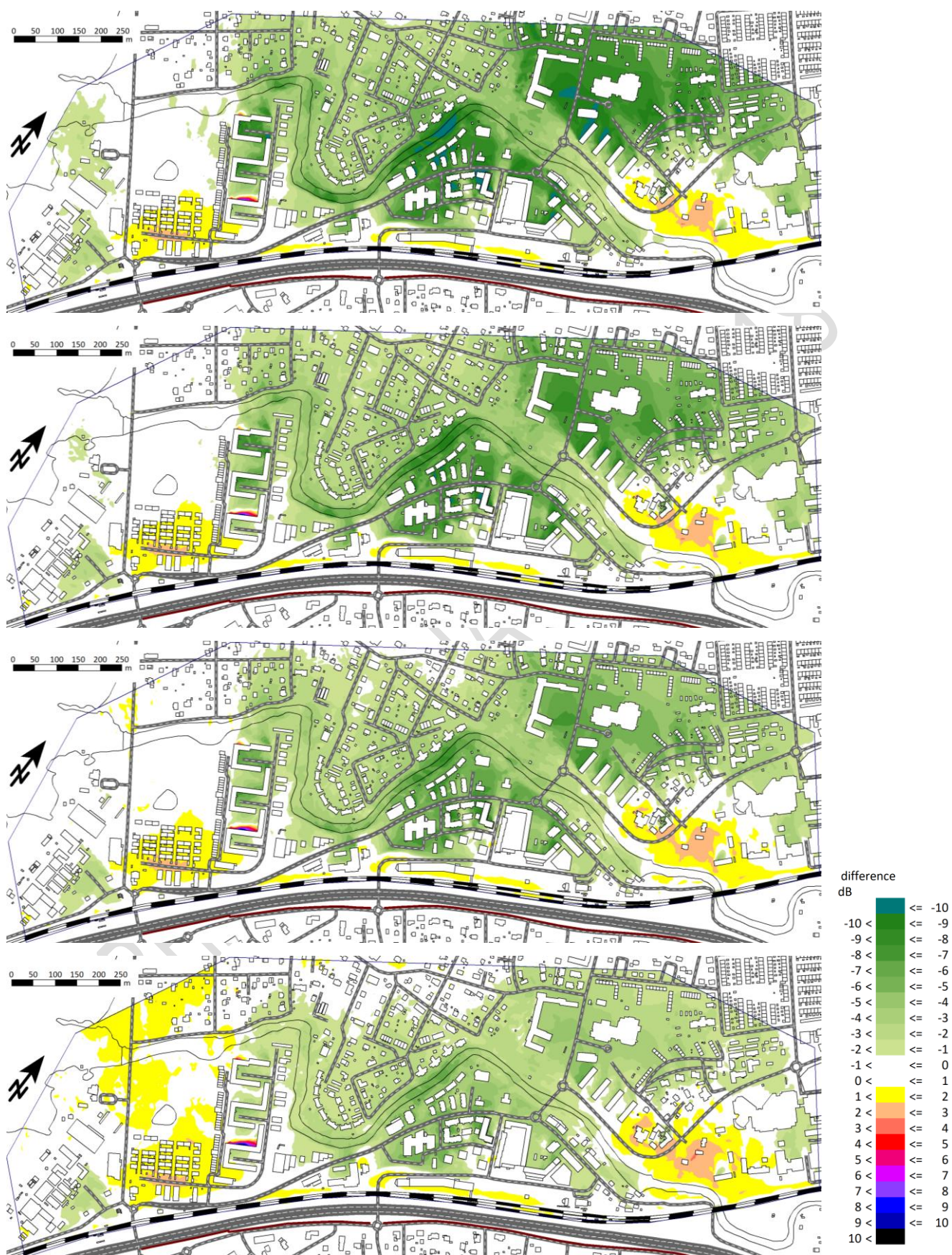
Figur 34. Lerum, centrum, skillnadsplottar (L Aeq24h ) Nord2000 – Nord96, beräkningshöjd = 8 m. Vindhastighet uppifrån: 1 m/s, 1,5 m/s, 2 m/s och 3 m/s.
