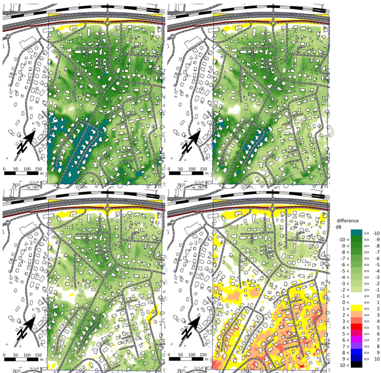
Figur 42. Lerum, villaområde, skillnadsplottar ( L_{AFmax} ) Nord2000 – Nord96, beräkningshöjd = 5 m.
