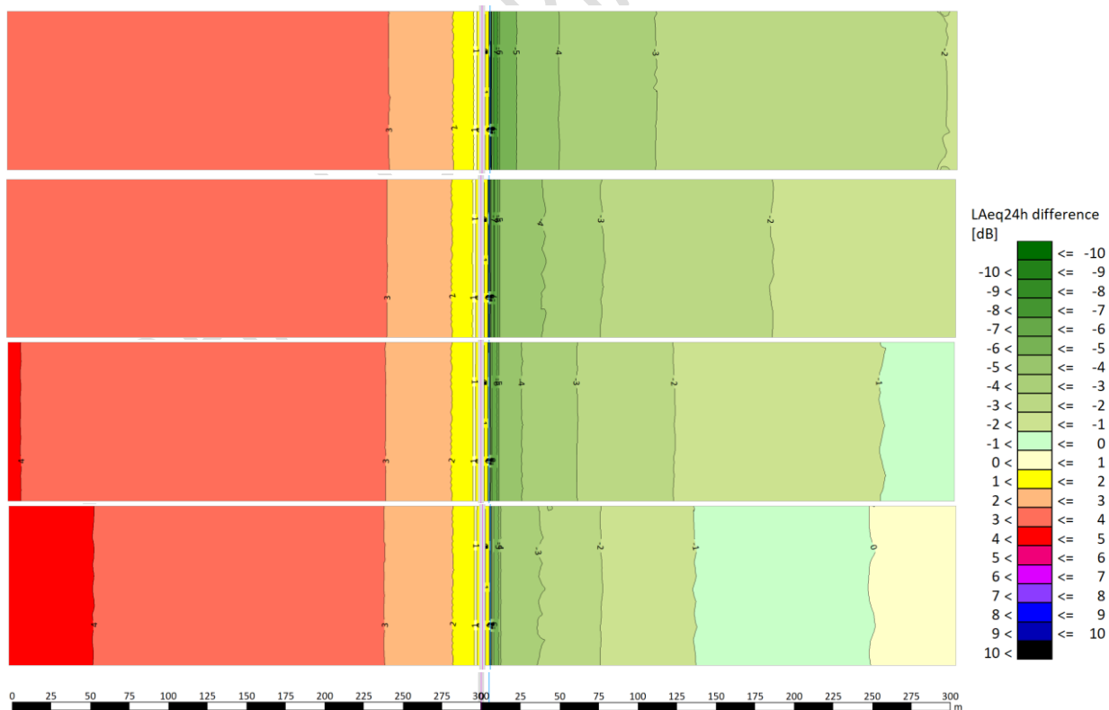
Figur 12. Skillnadsplottar ( L_{Aeq24h} ) Nord2000 – Nord96, beräkningshöjd = 2 m, höjd banvall = 2 m, mjuk mark. Vindhastighet uppifrån: 1 m/s, 1,5 m/s, 2 m/s och 3 m/s.
