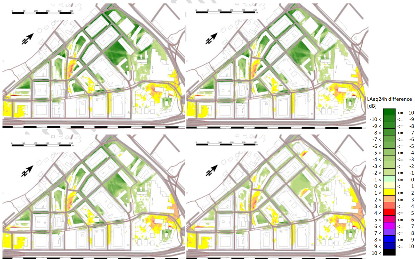
Figur 28. Brämaregården, skillnadsplottar ( L_{Aeq24h} ) Nord2000 – Nord96, beräkningshöjd = 8 m. Vindhastigheter: övre vänster 1 m/s, övre höger 1,5 m/s, nedre vänster 2 m/s och nedre höger 3 m/s.
