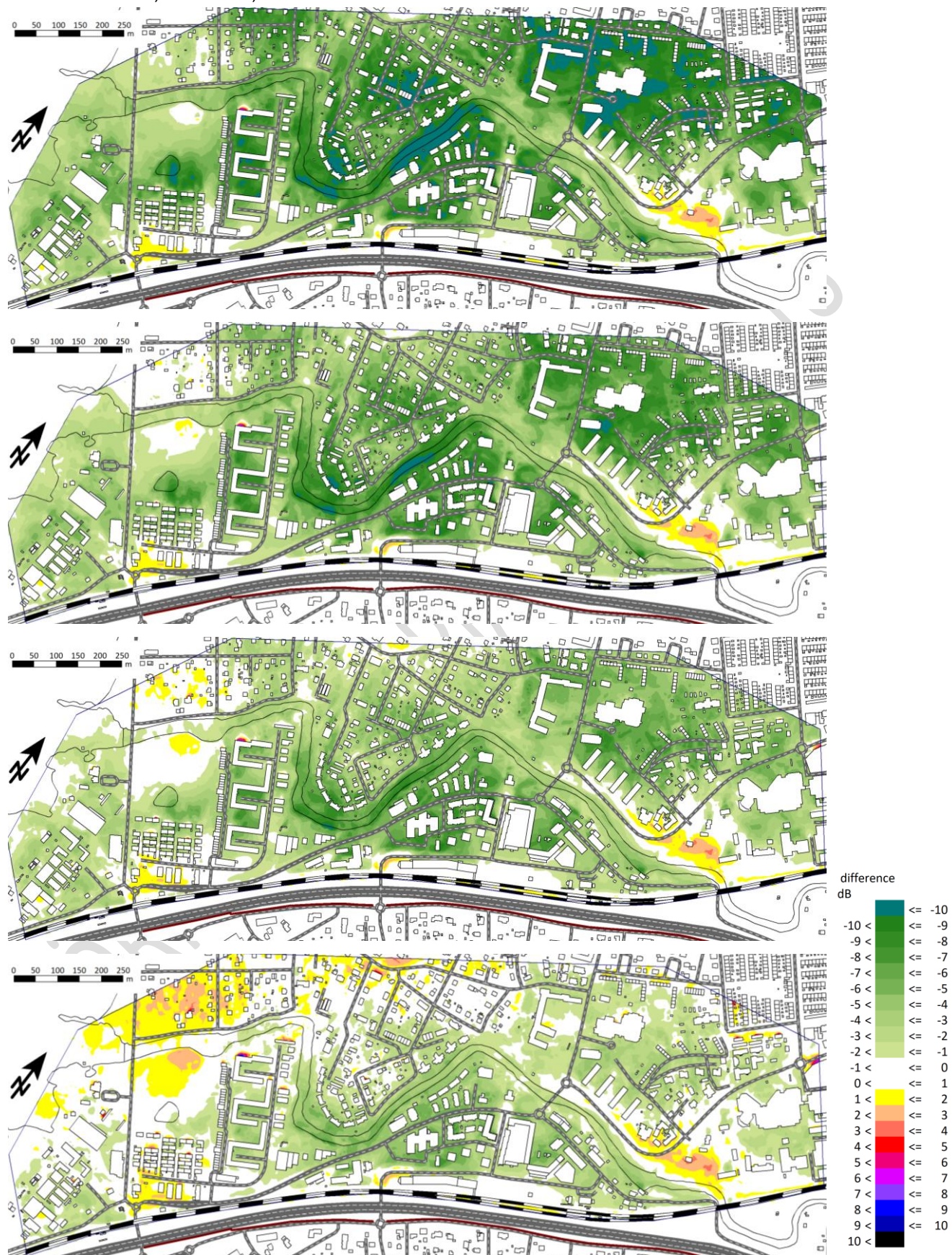
Figur 32. Lerum, centrum, skillnadsplottar ( L_{Aeq24h} ) Nord2000 – Nord96, beräkningshöjd = 2 m. Vindhastighet uppifrån: 1 m/s, 1,5 m/s, 2 m/s och 3 m/s.
