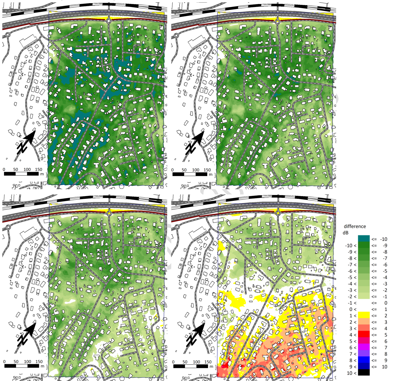
Figur 38. Lerum, villaområde, skillnadsplottar ( L_{Aeq24h} ) Nord2000 – Nord96, beräkningshöjd = 2 m. Vindhastigheter: övre vänster 1 m/s, övre höger 1,5 m/s, nedre vänster 2 m/s och nedre höger 3 m/s.
